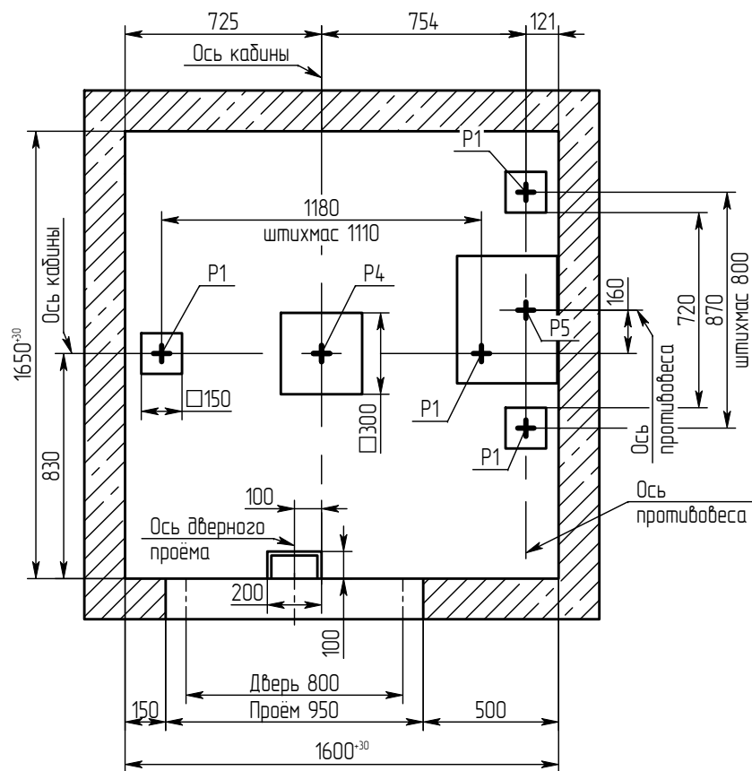
Б – Б (1:25) (1)
